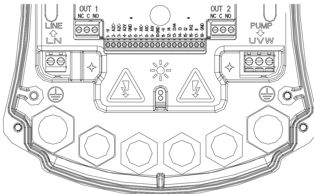
Схема 1: Электропроводка
